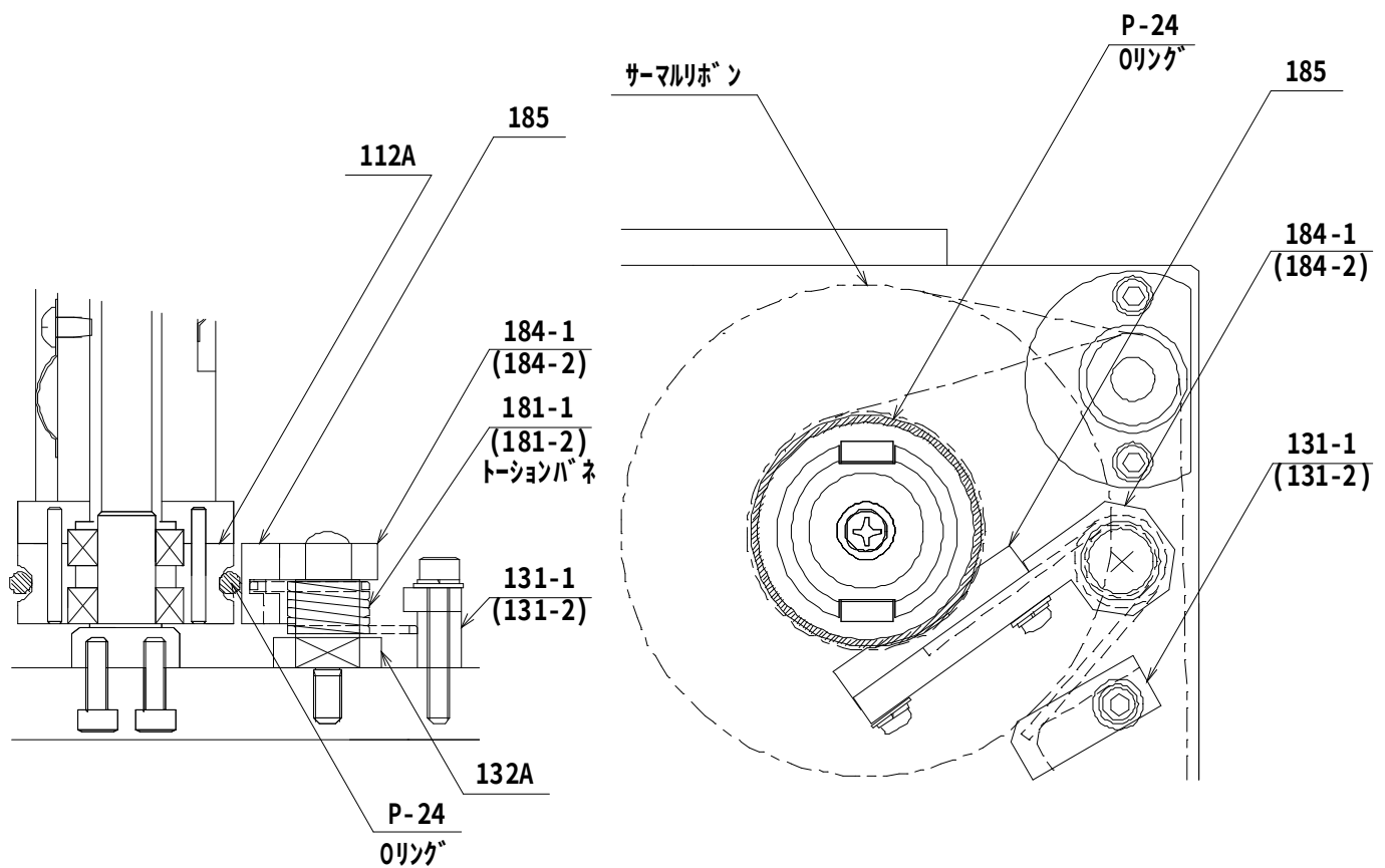
供給リールとリボンエンコーダ
