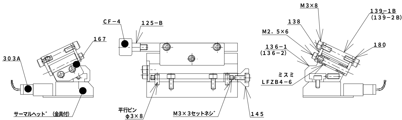
サーマルヘッド詳細
