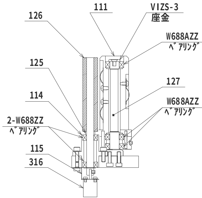
供給リールとリボンエンコーダ
