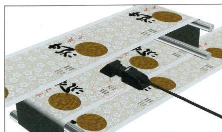
狭いところでの文字認識
